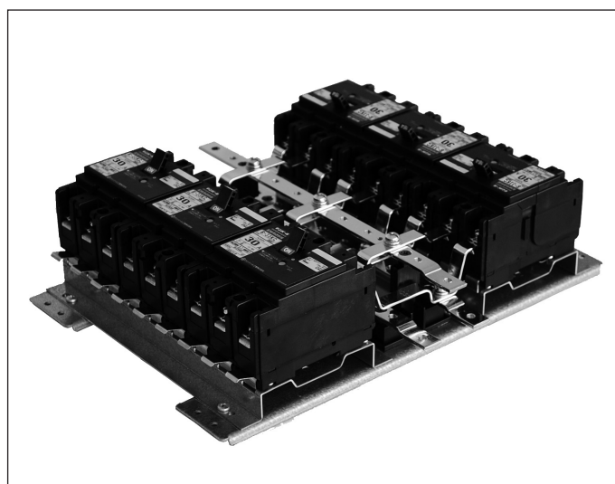
分電盤協約形サイズ配線用遮断器分岐ユニット
