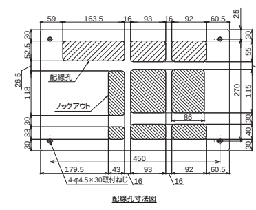
配線孔寸法図
