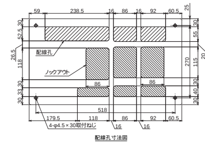
配線孔寸法図
