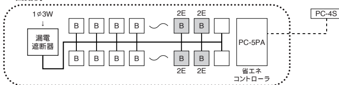
回路例
