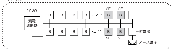
回路例
