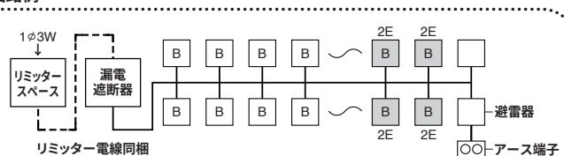
回路例
