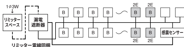
回路例
