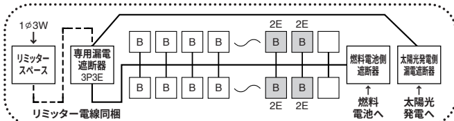
回路例
