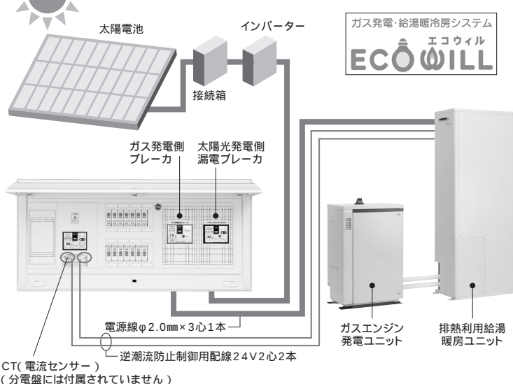
家庭用ガス発電・給湯暖房機 + 太陽光発電システム用電気系統接続概要図
