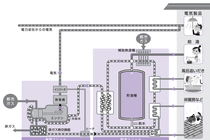
家庭用ガス発電・給湯暖房機のしくみと熱の利用先
