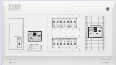
太陽光側遮断器 BU-53・1ECS(50AF/30AT)
