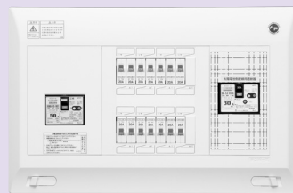
太陽光側遮断器 BU-53・1ECS(50AF/30AT)
