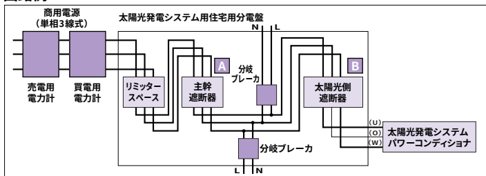
回路例1
