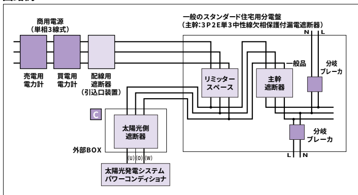
回路例2
