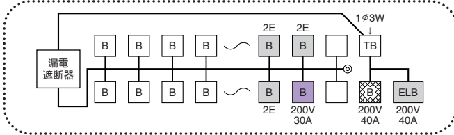
回路例
