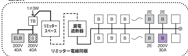
回路例
