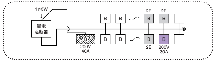
回路例
