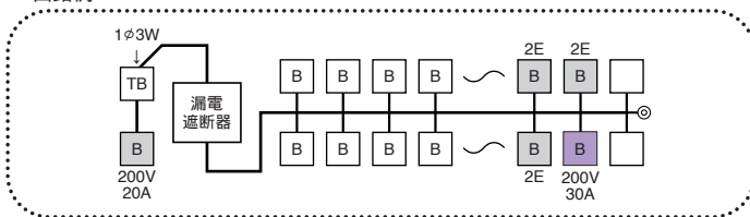
回路例
