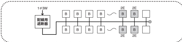
回路例
