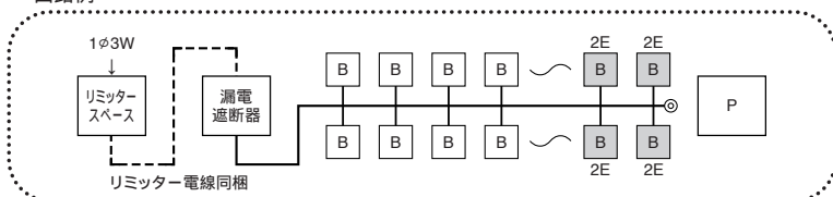
回路例
