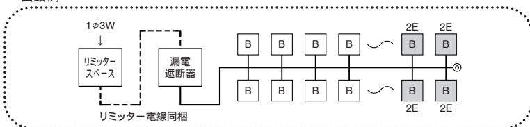
回路例
