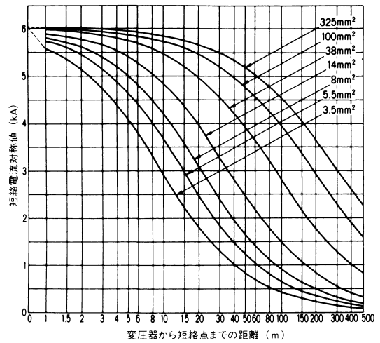
付図9 三相変圧器容量150kVA、二次電圧415V
