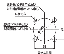
パネル穴明加工図
