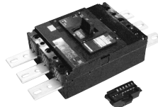
カセット付属装置 警報スイッチユニット(AL) カセット付属装置 補助スイッチユニット(AX)
