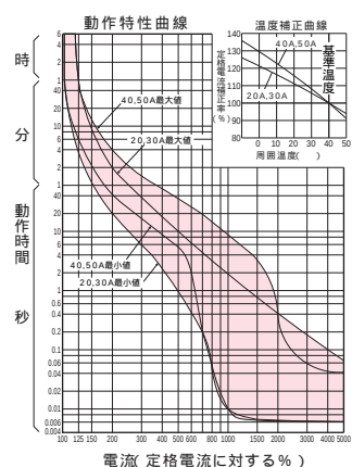
GBU-53・1KC、GBU-53・1KCS、GBU-53KC
