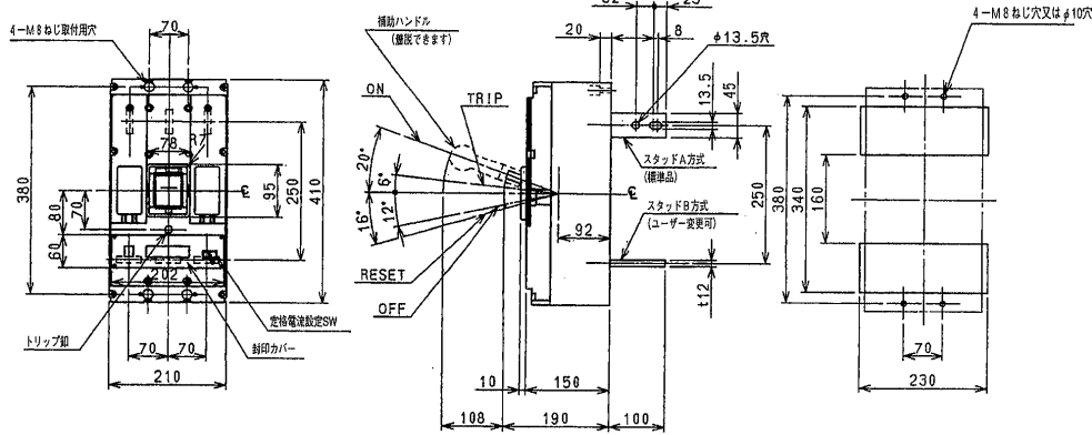
埋込形(FP)
