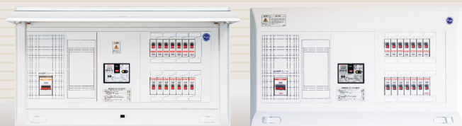
エコキュート・電気温水器＋ IHクッキングヒーター
