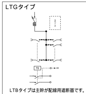
LTBタイプは主幹が配線用遮断器です。
