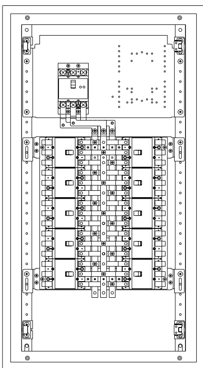
分岐：協約形配線用遮断器（3P）
