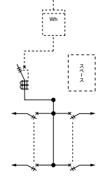
LWCBタイプは主幹が配線用遮断器です。
