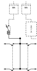
LW2CBタイプは主幹が配線用遮断器です。
