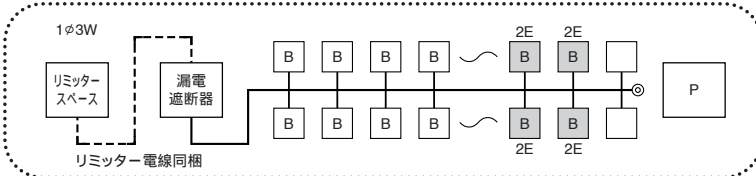
回路例
