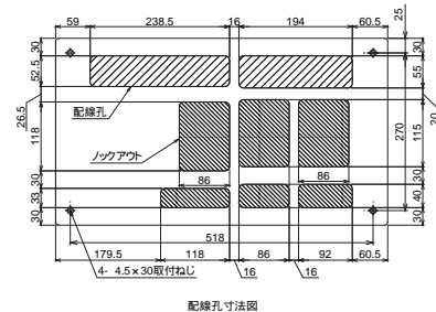
配線孔寸法図
