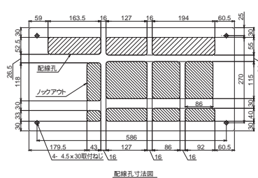
配線孔寸法図
