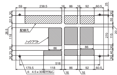
配線孔寸法図
