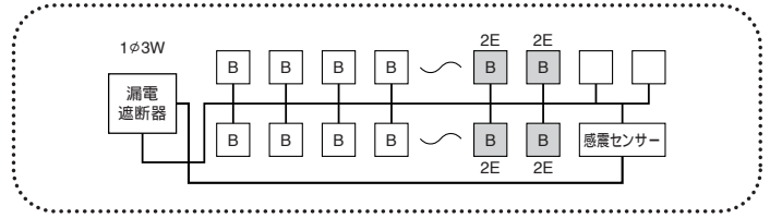
回路例
