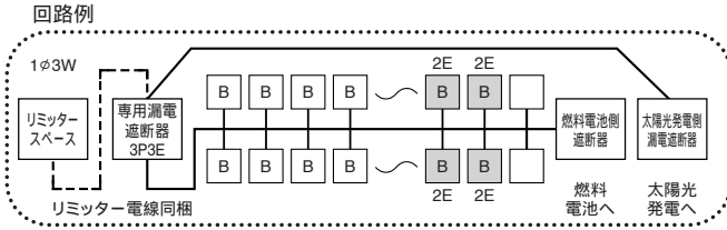
燃料電池側遮断器 B-33EC(30AF/20AT)
