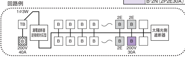
太陽光側遮断器 単3連系の場合 B-53EC(50AF/30AT) 単2連系の場合 BU-53・1ECS(50AF/30AT)
