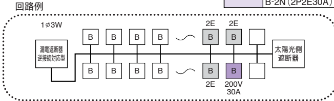
太陽光側遮断器
