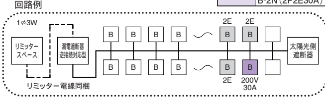
太陽光側遮断器 単3連系の場合 B-53EC(50AF/30AT) 単2連系の場合 BU-53・1ECS(50AF/30AT)
