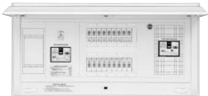
太陽光発電システム対応遮断器組込例
