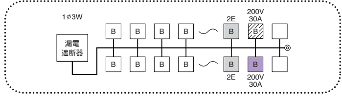
回路例
