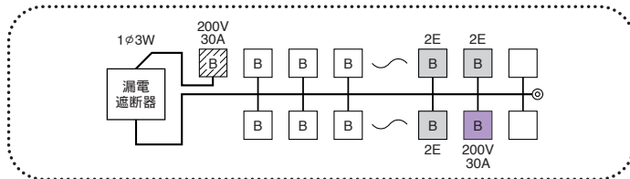
回路例
