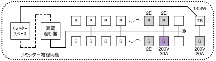
回路例
