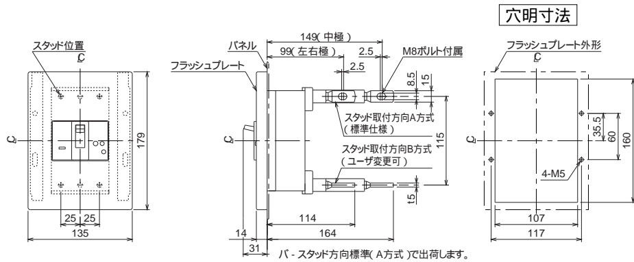
GB-102EC, GB-103EC
