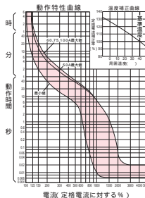
GB-102EC, GB-103EC
