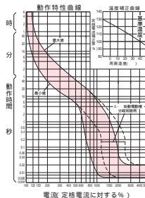
GB-152EC, GB-153EC
