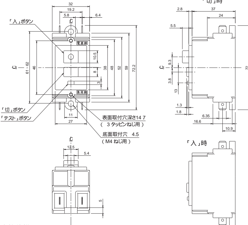
機器表面取付例
