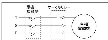
単相電動機への結線方法
