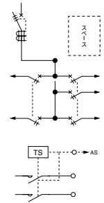
LTBタイプは主幹が配線用遮断器です。
