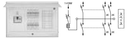
付属機器取付スペース付 タテ ヨコ フカサ 175 x 75 x 48
