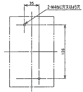
穴明寸法
