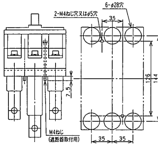
穴明寸法
