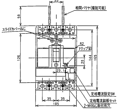
裏面形 (SD)
