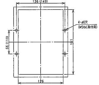
穴明寸法
