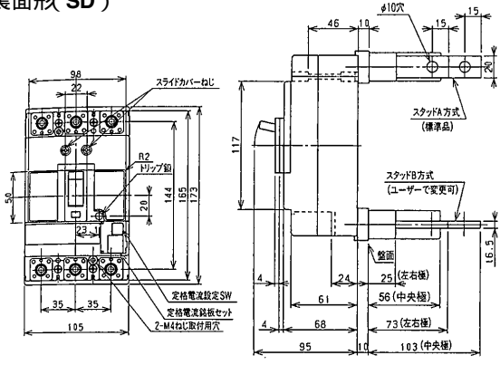
裏面形 (SD)
