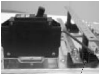
ミニ・イコールブレーカ 200V切替バー (ULK033片側) (ULK035両側)
