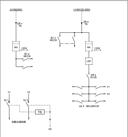
■ 回路図 (B)
