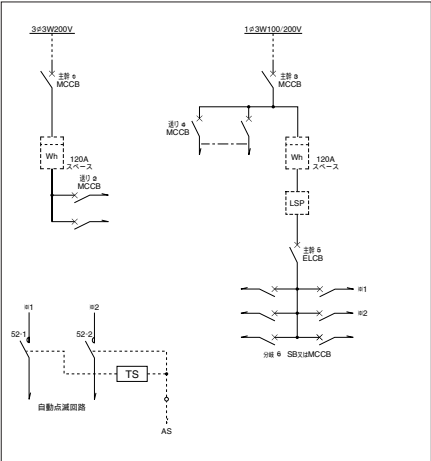
■ 回路図 (A)
