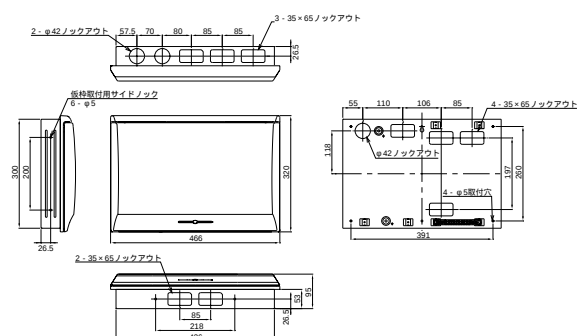
埋込形
