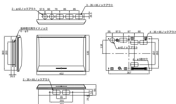
埋込形
