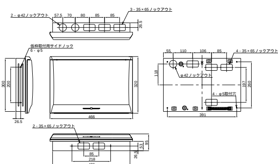
埋込形
