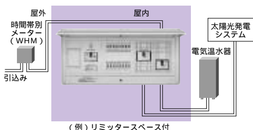
太陽光発電システム + 時間帯別電灯契約用住宅用分電盤 使用時の施工方法
