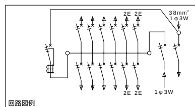
組込例
